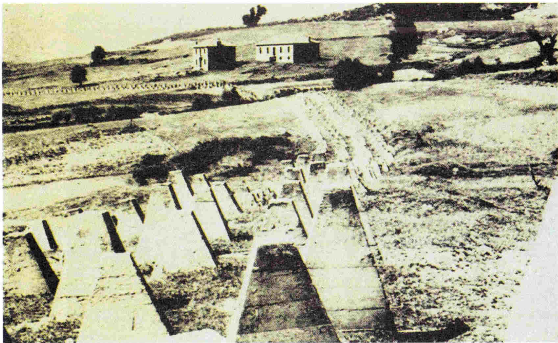
«Γραμμή Μεταξᾶ». Αντιαρματικά ἐμπόδια, κατασκευασμένα εἰς τοποθεσίας, ἐκ τῶν ὁποίων ἦτο πιθανὸν νὰ περάσουν ἄρματα μάχης.
