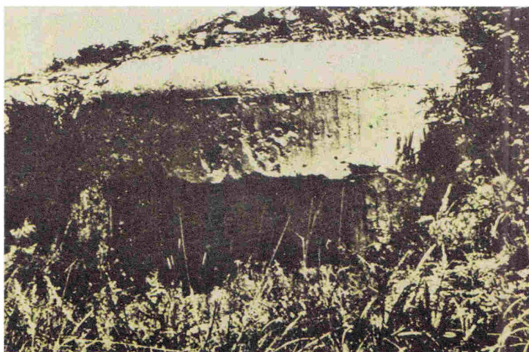
Φάτνωμα πολυβολείου τῆς «Γραμμῆς Μεταξᾶ». Τὰ ἐχθρικὰ βλήματα ἔχουν ἀφήσει ἵχνη εἰς τὸ τσιμέντο.
