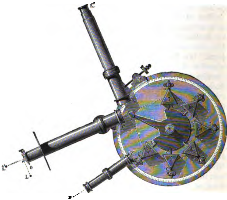
FIG. 143.—SPECTROSCOPE
