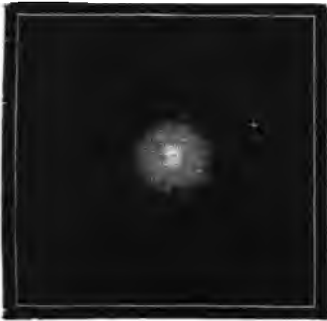
FIG. 25.—NEBULA : PRIMORDIAL CONDENSATION
