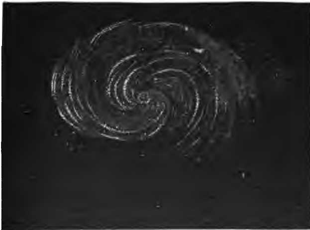
FIG. 282.—SPIRAL NEBULA IN CANES VENATICI
